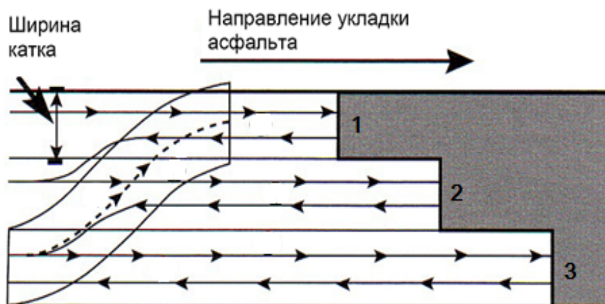
Рисунок 9 – Схема движения катка
