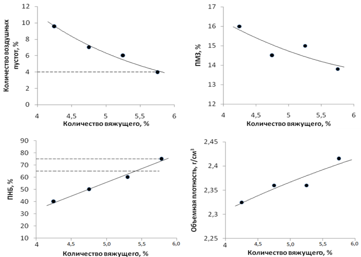
Рисунок 3 – Примеры зависимостей объемных свойств
