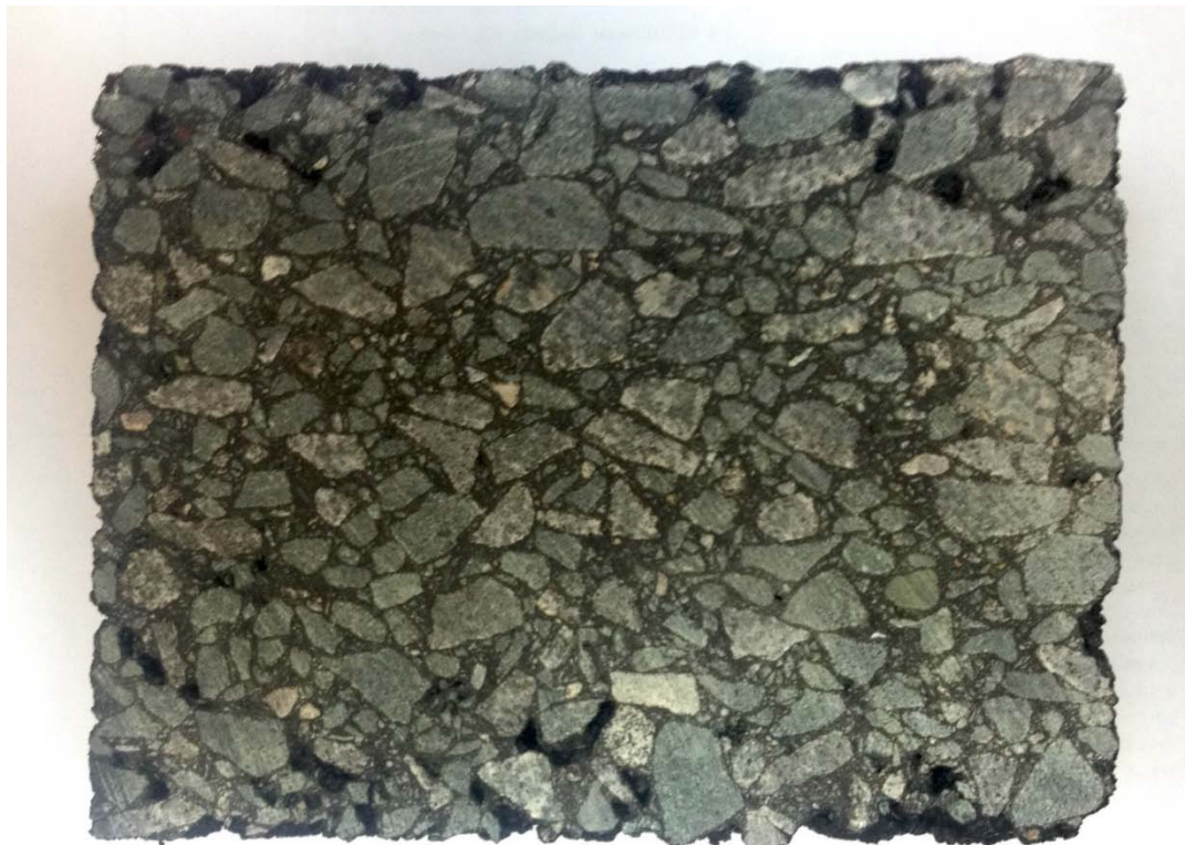
Рисунок А.9– Поверхность разреза асфальтобетонного образца SP-19
