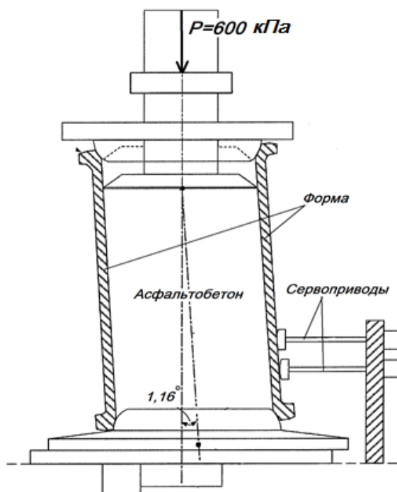
Рисунок 2 – Принцип работы вращательного уплотнителя (гиратора)
