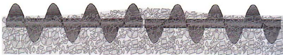
Рисунок 8 – Правильный уровень смеси, переносимой в камере шнека асфальтоукладчика
