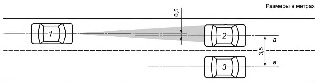
1 — управляемый автомобиль; 2 — впереди идущий автомобиль на пути следования управляемого автомобиля; 3 — впереди идущий автомобиль на соседней полосе; а — скорость каждого автомобиля, равная V_{\text{vehicle\_start}}
