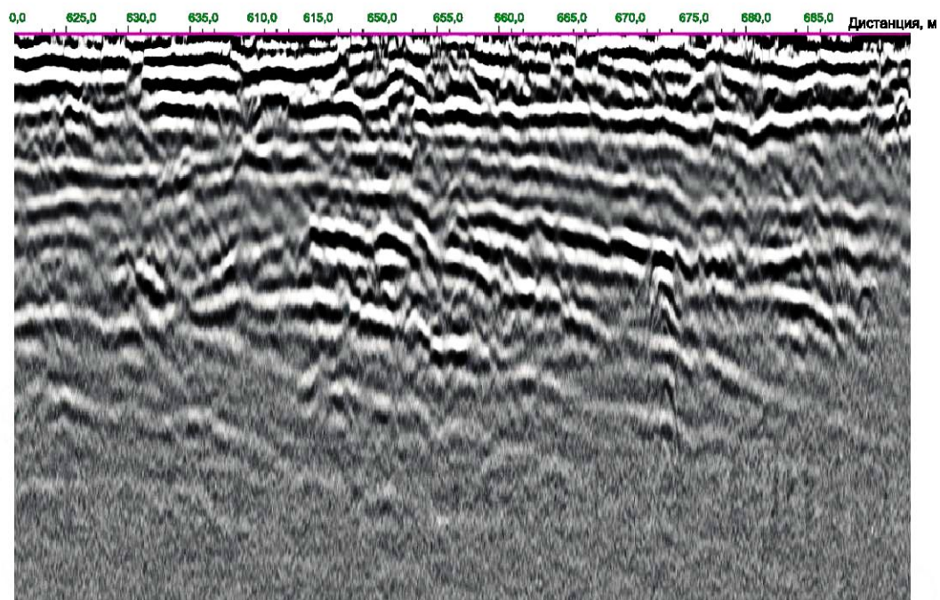
Рисунок Г.3 — Тип записи линзовидный, косослоистый — характерен для песчаных и супесчаных насыпей с неравномерным уплотнением (внутри каждого слоя преобладает прозрачный тип записи)
