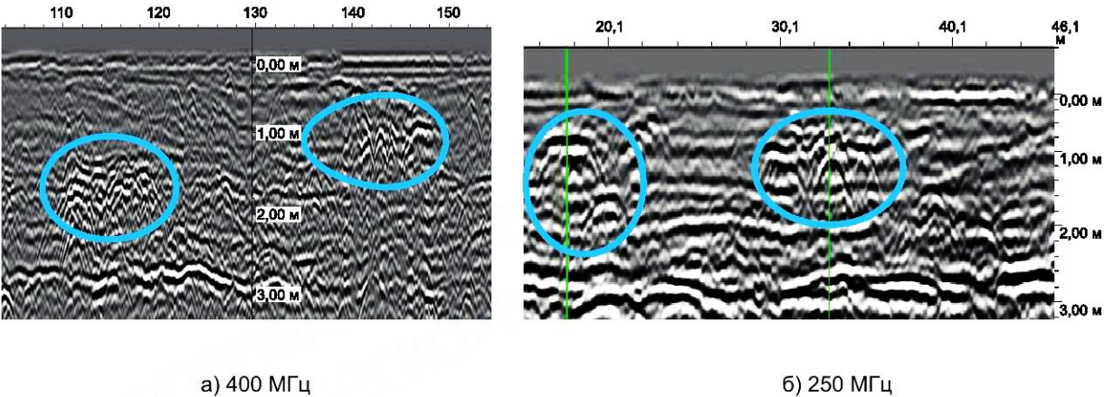
Рисунок 7.1 — Фрагменты радарограмм с выделенными скоплениями мерзлых комьев
