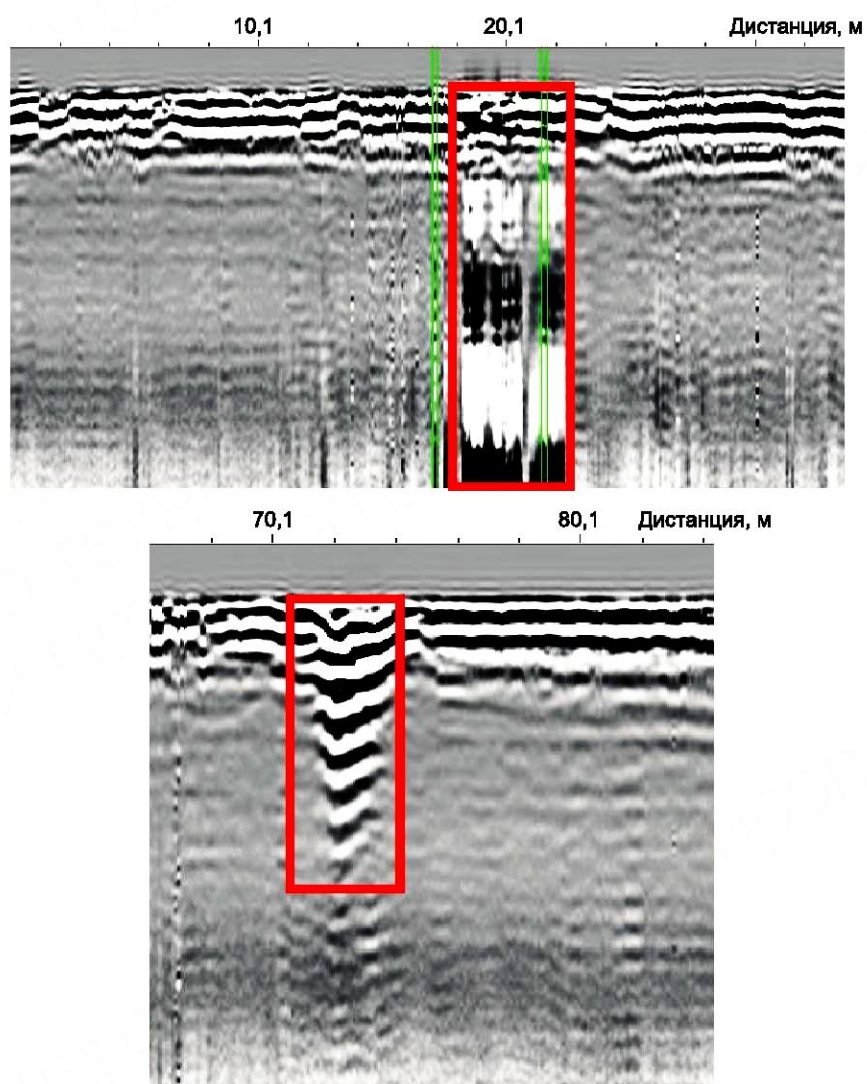
Рисунок Г.6 — Тип записи «звонящий» (многократные переотражения сигнала) — характерен для переувлажненных грунтов
