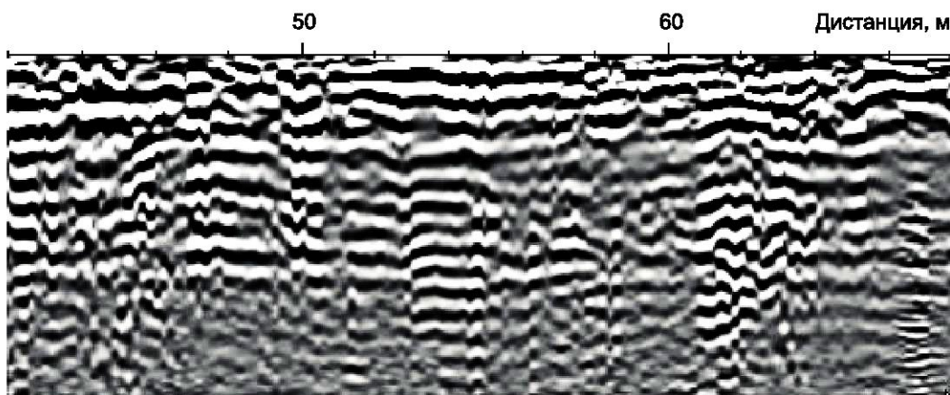
Рисунок Г.5 — Тип записи параллельно-слоистый — характерен для песчаных и супесчаных насыпных грунтов при послойном уплотнении
