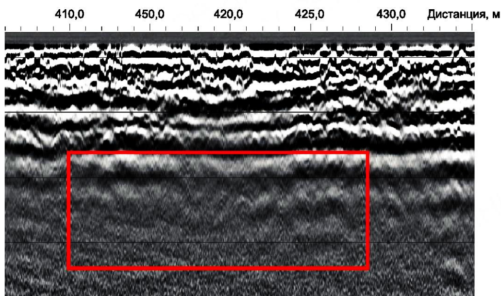
Рисунок Г.2 — Тип записи затухающий, прозрачный — характерен для суглинистых грунтов
