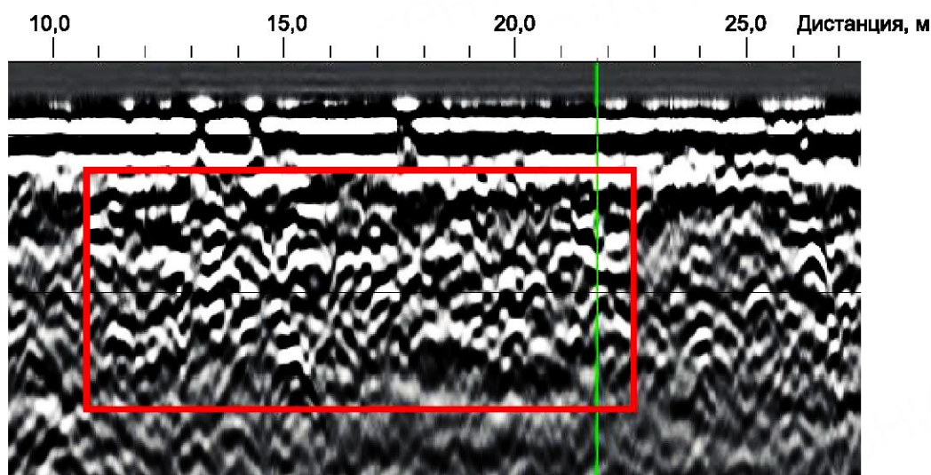
Рисунок Г.1 — Тип записи хаотичный — характерен для крупнообломочного грунта
