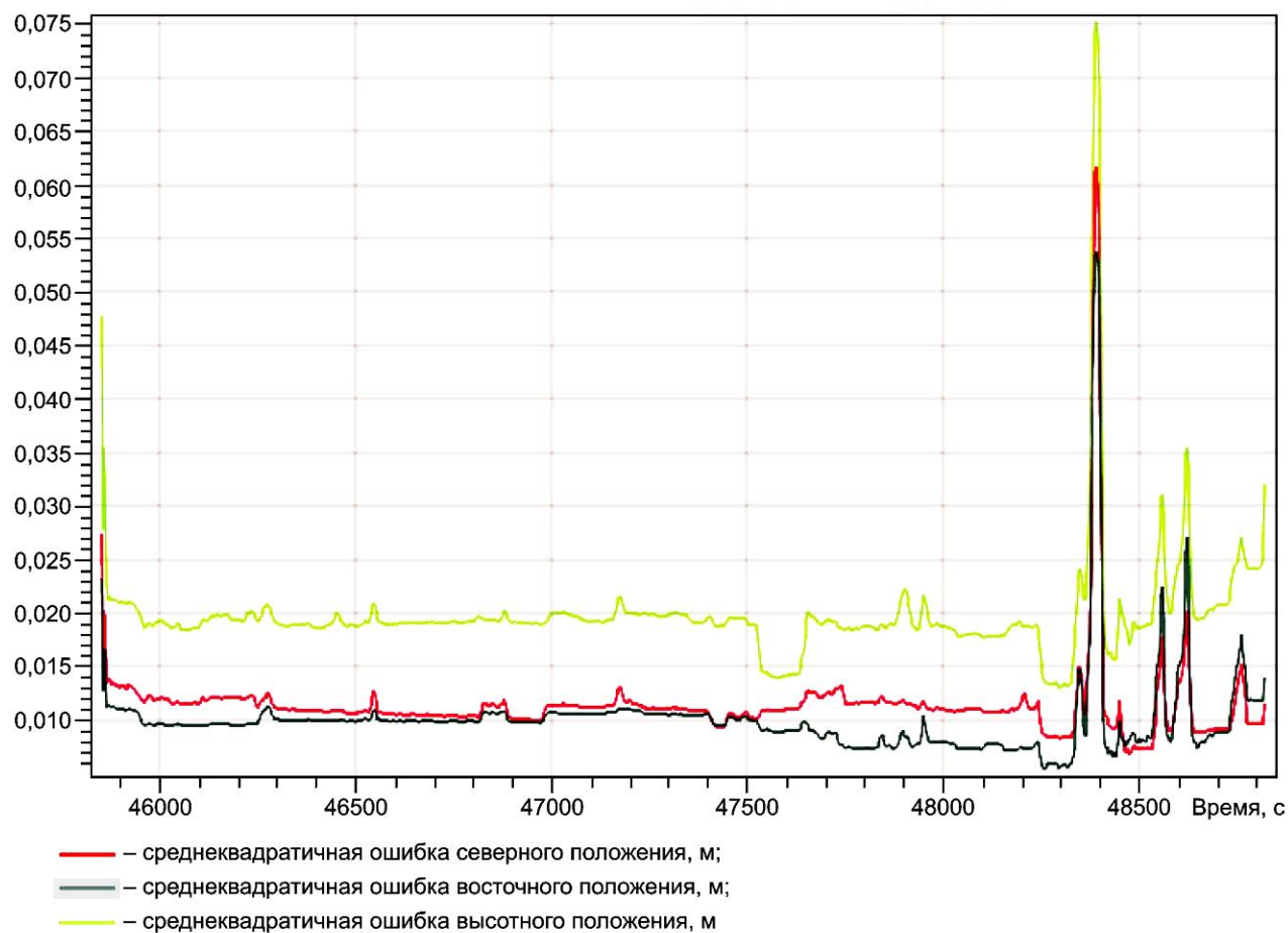
Рисунок А.1 — Форма результата оценки точности траекторий движения системы лазерного сканирования
