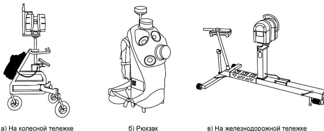
Рисунок 2 — Варианты монтажа мобильных систем лазерного сканирования на немоторизованных платформах
