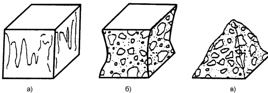
Рисунок 7.3 — Удовлетворительное разрушение образцов-кубов
