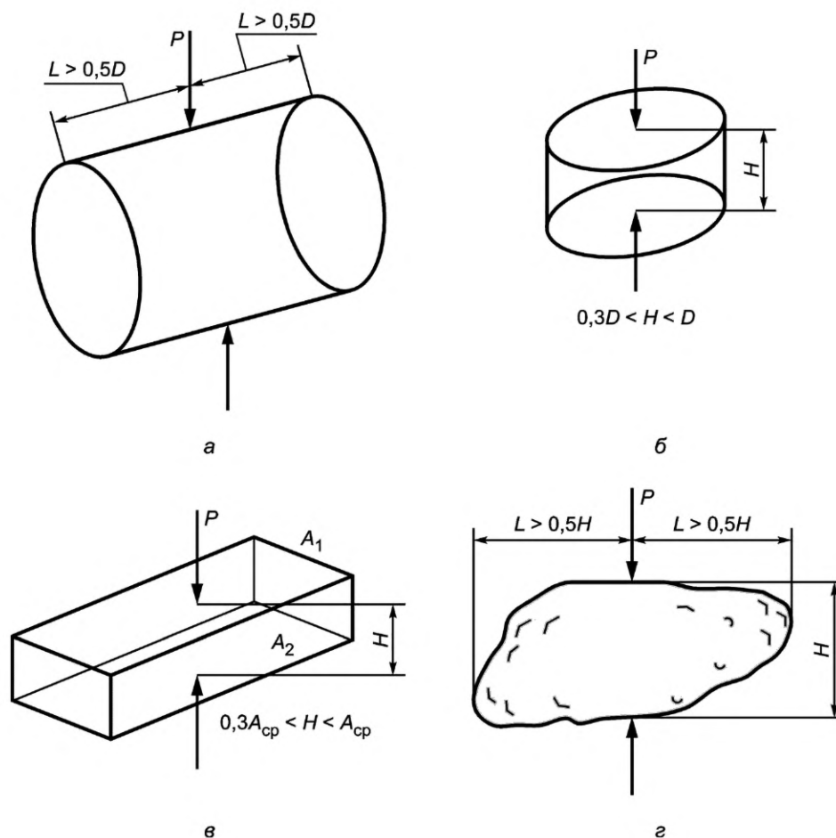
а — горизонтальный цилиндрический образец; б — вертикальный цилиндрический образец; в — образец в форме прямоугольного параллелепипеда; г — образец неправильной формы
