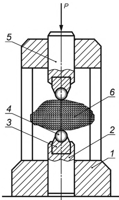
1 — силовая рама; 2 — нижний шток либо основание; 3, 4 — вкладыш со сферическим индентором или конусный индентор; 5 — верхний шток; 6 — образец
