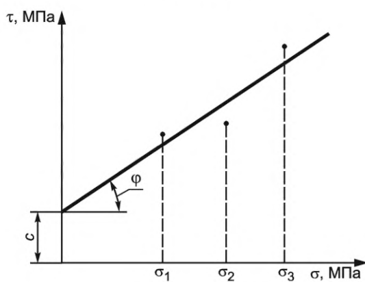
Рисунок Г.2 — График \tau = f(\sigma)
