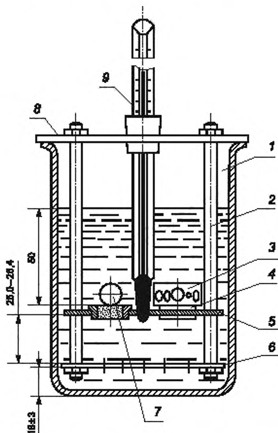
1 — стеклянный стакан; 2 — штатив; 3 — накладка; 4 — латунное ступенчатое кольцо; 5 — верхняя пластинка; 6 — нижняя пластинка; 7 — шарик; 8 — крышка; 9 — термометр
