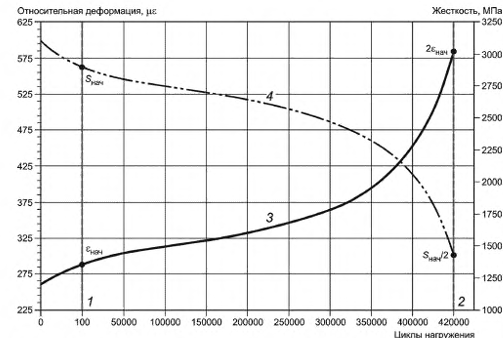
1 — начальная относительная деформация и начальная жесткость (на сотом цикле нагружения); 2 — момент разрушения N_R ; 3 — развитие относительной деформации в испытуемом образце; 4 — падение жесткости испытуемого образца
