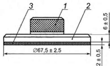
1 — рукоятка; 2 — диск; 3 — резиновое покрытие
