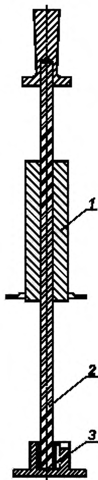
1 — скользящий груз, 2 — стержень; 3 — пружина
