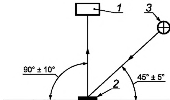
1 — спектрофотометр или колориметр, для измерения коэффициента яркости применяется яркомер; 2 — полимерная лента; 3 — источник света
