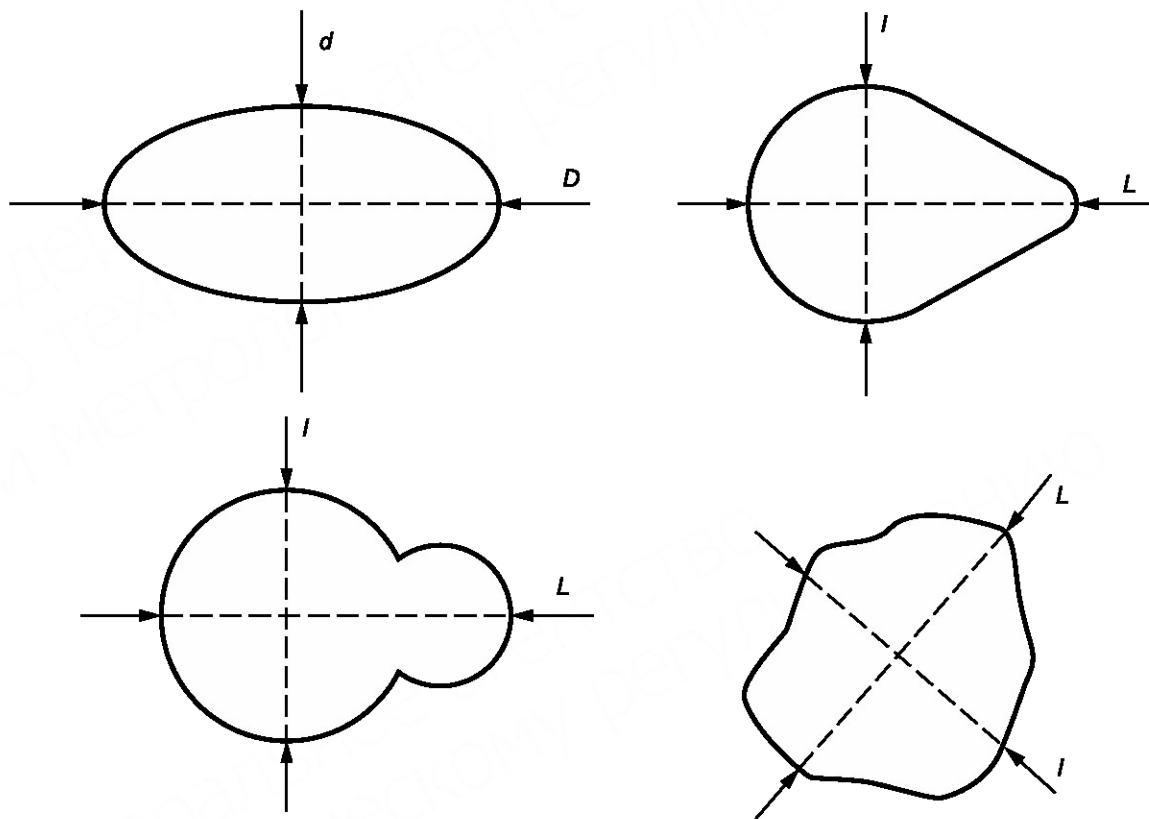
Рисунок Б.1 — МСШ некруглой формы
