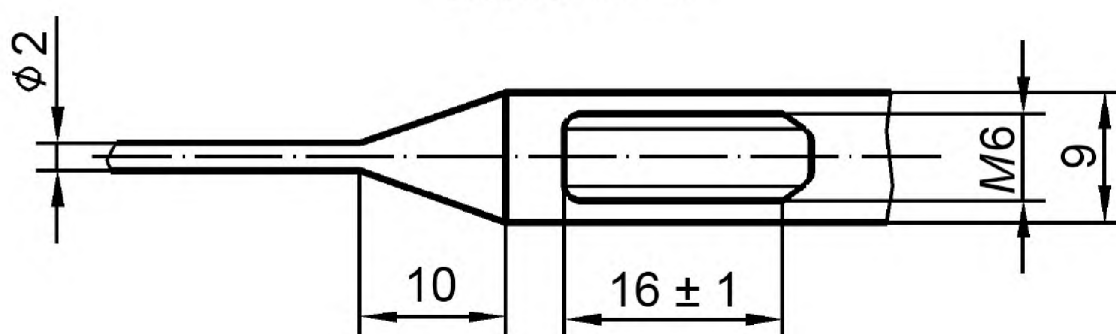
Рисунок 5 – Зажимы
