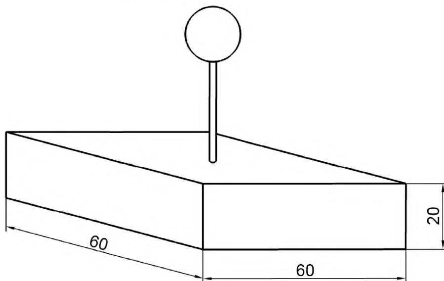
Рисунок 2 – Металлическая крышка (толщина листа – 1,5 мм)
