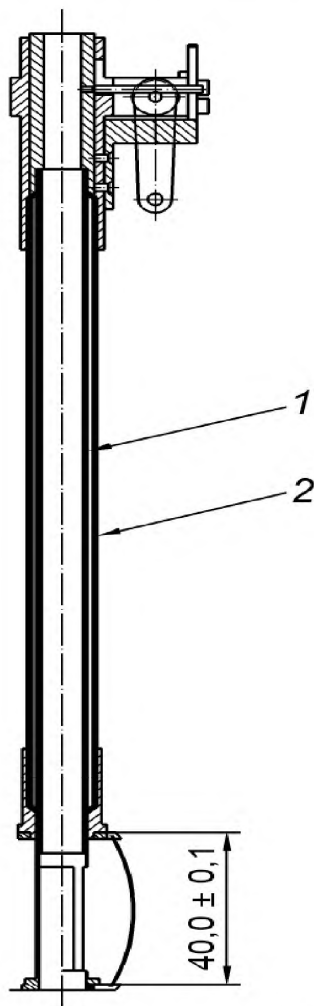
1 – внутренняя трубка изгибающего устройства наружным диаметром 11,5 мм и внутренним диаметром 7,5 мм; 2 – наружная трубка изгибающего устройства наружным диаметром 16,5 мм, внутренним диаметром 12,5 мм
