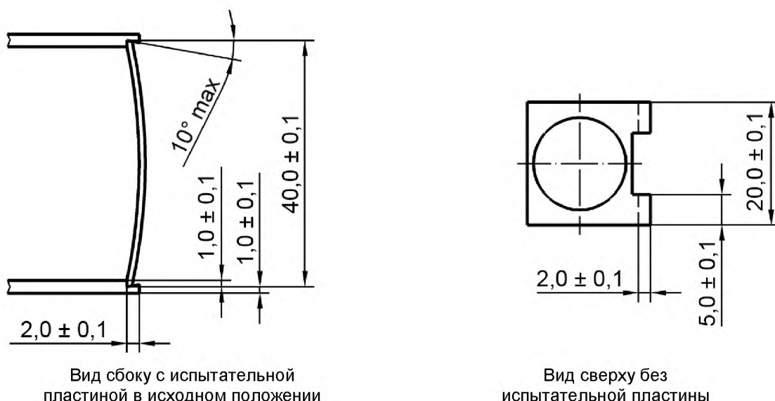
Рисунок 5 – Зажимы
