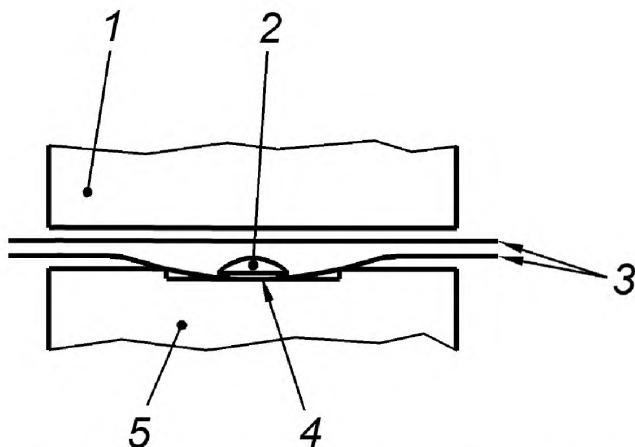
1 – верхний прижимной брусок; 2 – проба; 3 – разделительная пленка; 4 – испытательная пластина; 5 – нижний прижимной брусок
