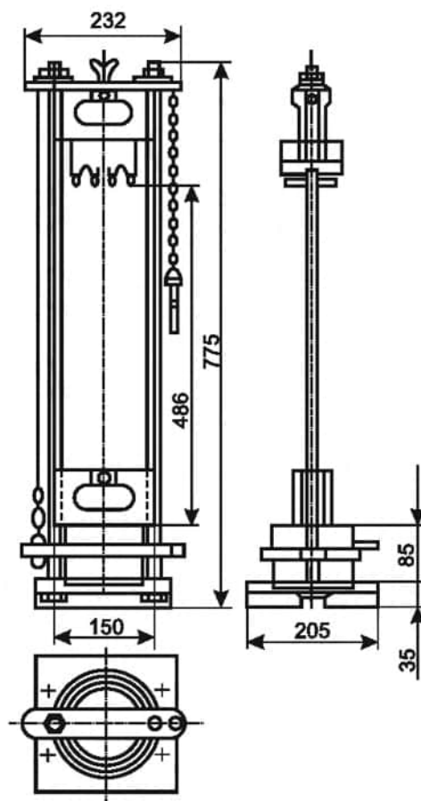
Рисунок 11 — Копер ПМ
