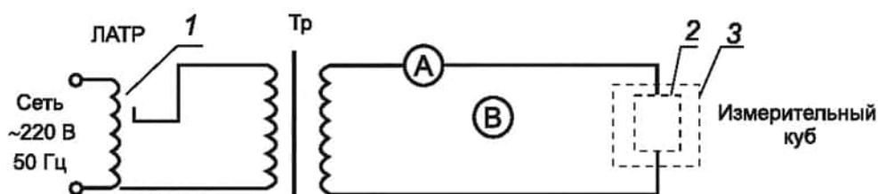
1 — лабораторный регулировочный трансформатор (ЛАТР); 2 — электрод; 3 — измерительный куб
