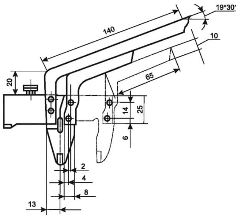
Рисунок 3 — Передвижной шаблон
