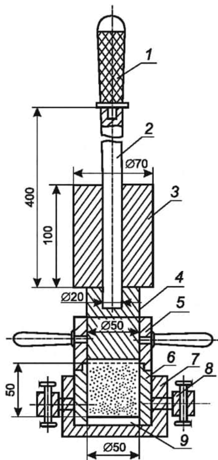
1 — рукоятка; 2 — направляющий стержень; 3 — гири; 4 — плунжер; 5 — направляющий насадный цилиндр; 6 — разъемный цилиндр; 7 — подстаканник; 8 — закрепляющие винты; 9 — металлическая пластинка
