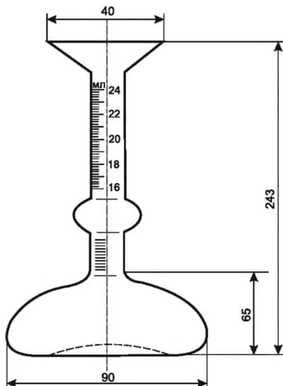
Рисунок 7 — Прибор Ле Шателье
