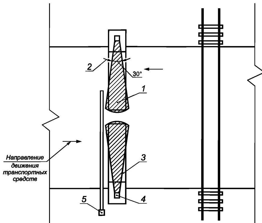
1 — диаграмма направленности; 2 — ширина диаграммы направленности; 3 — крышка ЗД; 4 — ЗЗК; 5 — шлагбаум
