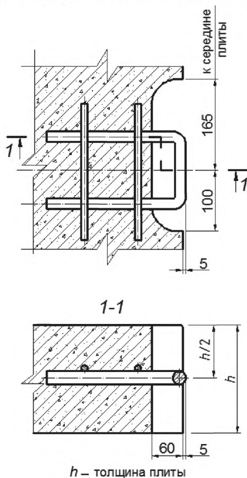
Рисунок 2 – Пример конструкции монтажно-стыкового соединения
