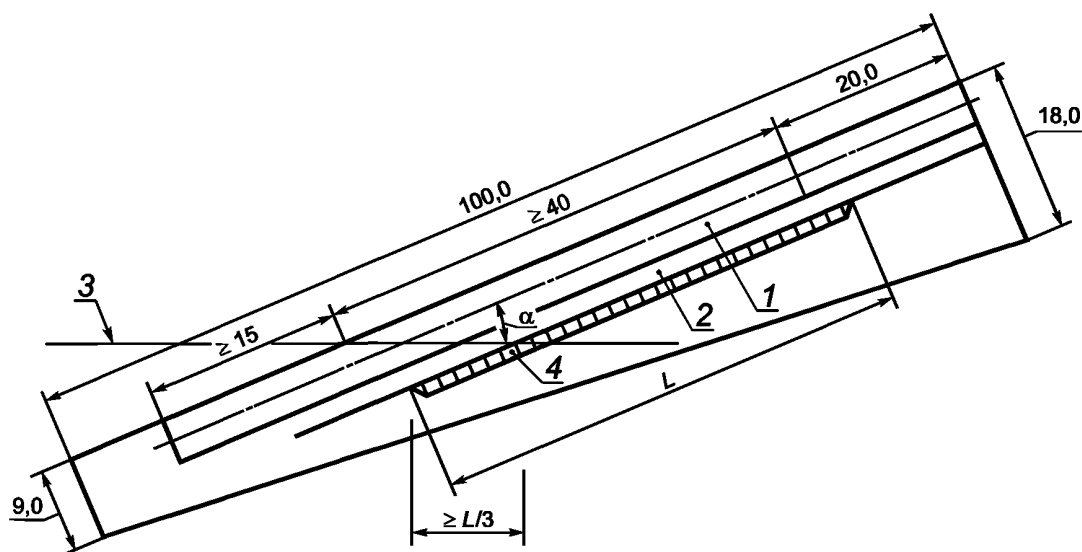
1 — полоса для испытаний ограждений мостовой группы; 2 — полоса для испытаний ограждений дорожной группы; 3 — ось направляющего монорельса для разгона испытательного автомобиля; 4 — установленное ограждение дорожной группы; L — длина ограждения; \alpha — угол удара
