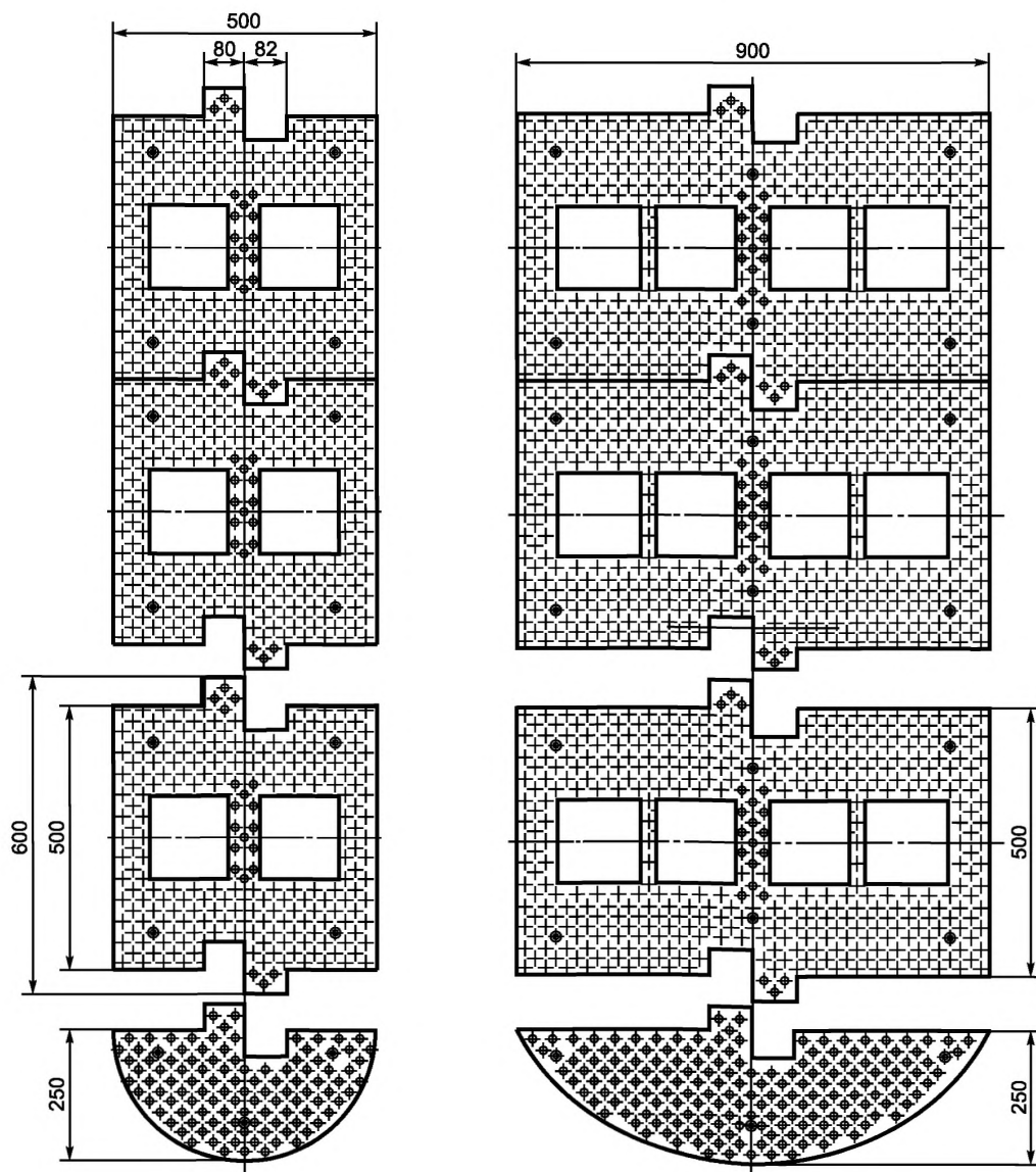
Рисунок Б.1 — Пример конструкции типовых ИНС
