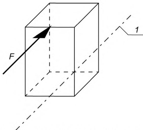
Рисунок 2 – Схема приложения нагрузки к тумбам класса ДТ2
