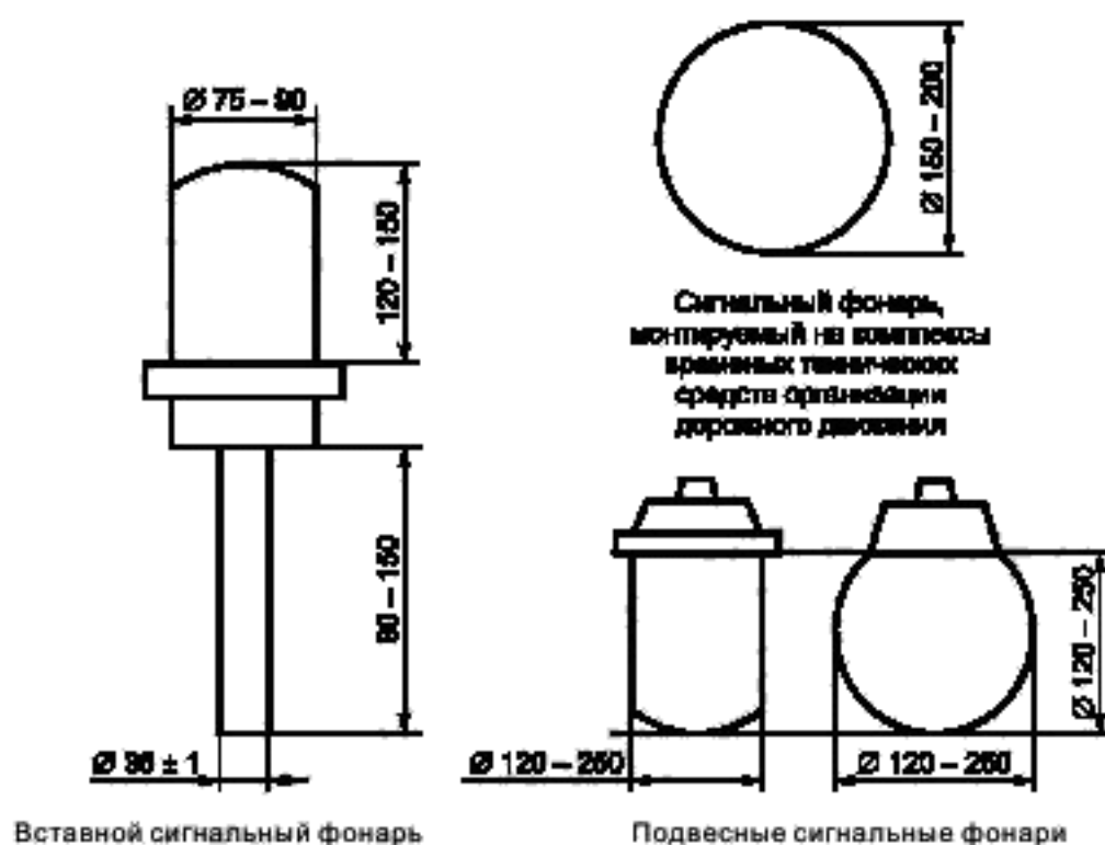
Рисунок 1 — Примеры схем сигнальных фонарей
