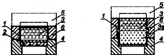
а) Форма типа I для приготовления образцов вида «грунт (грунтовый раствор, лед) — материал»
