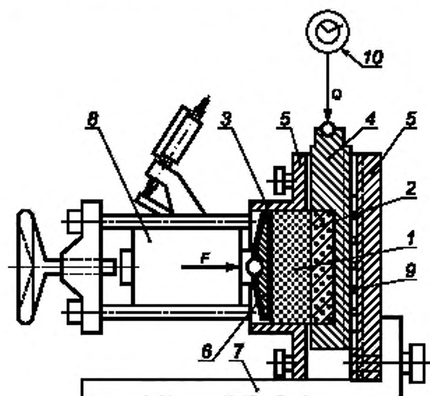
1 — мерзлый грунт; 2 — материал; 3 — рабочее кольцо; 4 — срезная каретка; 5 — корпус прибора; 6 — боковой штамп; 7 — опорная плита; 8 — динамометр; 9 — обойма шариков; 10 — мессура; Q — вертикальная нагрузка; F — горизонтальная нагрузка
