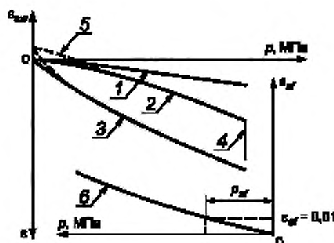
Рисунок В.1 — График 1, \varepsilon = f(p) по схеме «одной кривой»
