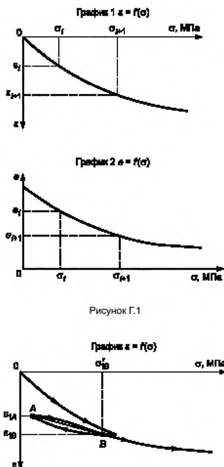
Рисунок Г.2 — График испытания методом компрессионного сжатия с определением модуля повторного нагружения
