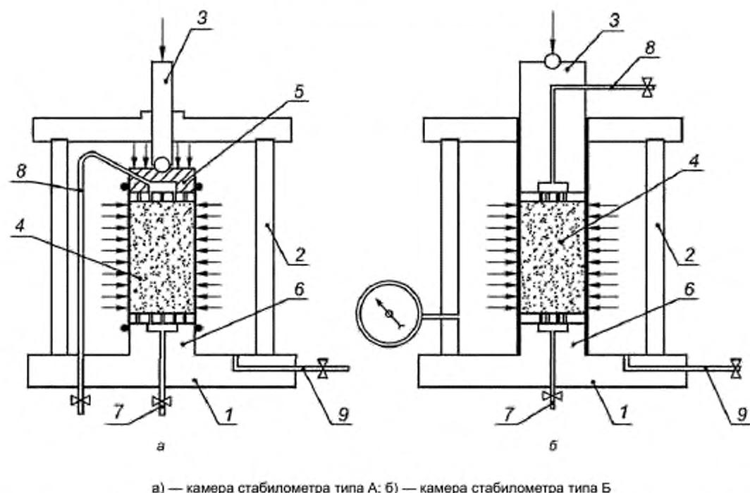
Рисунок Б.1 — Принципиальная схема камеры стабилометра для испытания грунта методом трехосного сжатия
